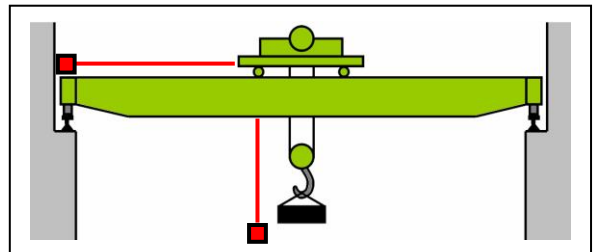
クレーンに荷重をかけての梁のタワミ測定、クレーンの位置調整
